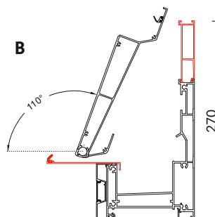
B. Wersja z dodatkową blendą wokół ramy maskująca widok lameli przy całkowitym otwarciu. Dopłata 60 EUR/mb obwodu
