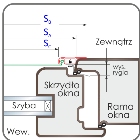
Ramka MINI na oknie
