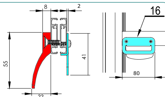
Skala 1:2
