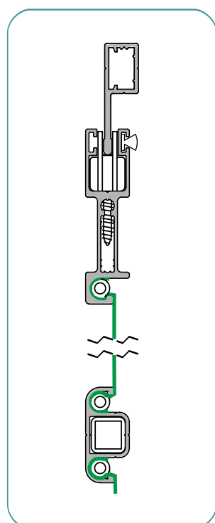
Montaż prowadnicy S III
