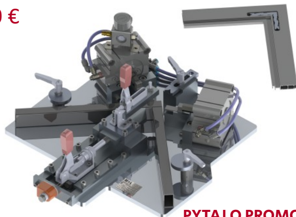
Zaciskarka do ram moskitier
