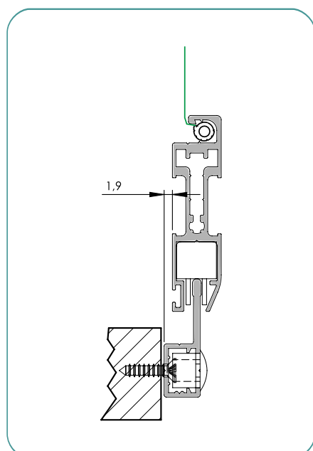
Montaż przewodnicy S III
