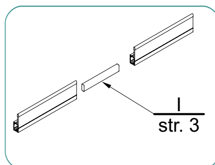
Łącznik prowadnicy S III
