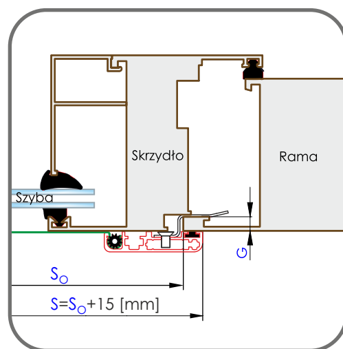
Ramka LICO w oknie
