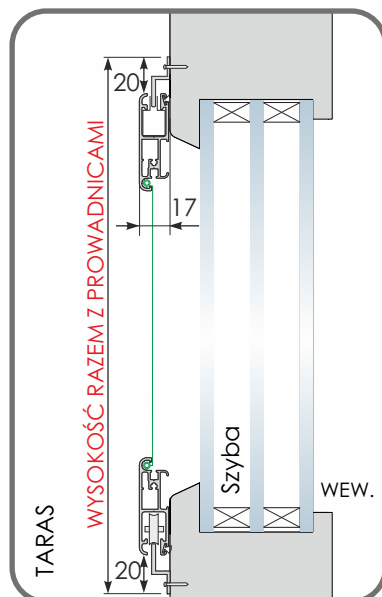
Prowadnica S II u góry i na dole do ramy [mm]
