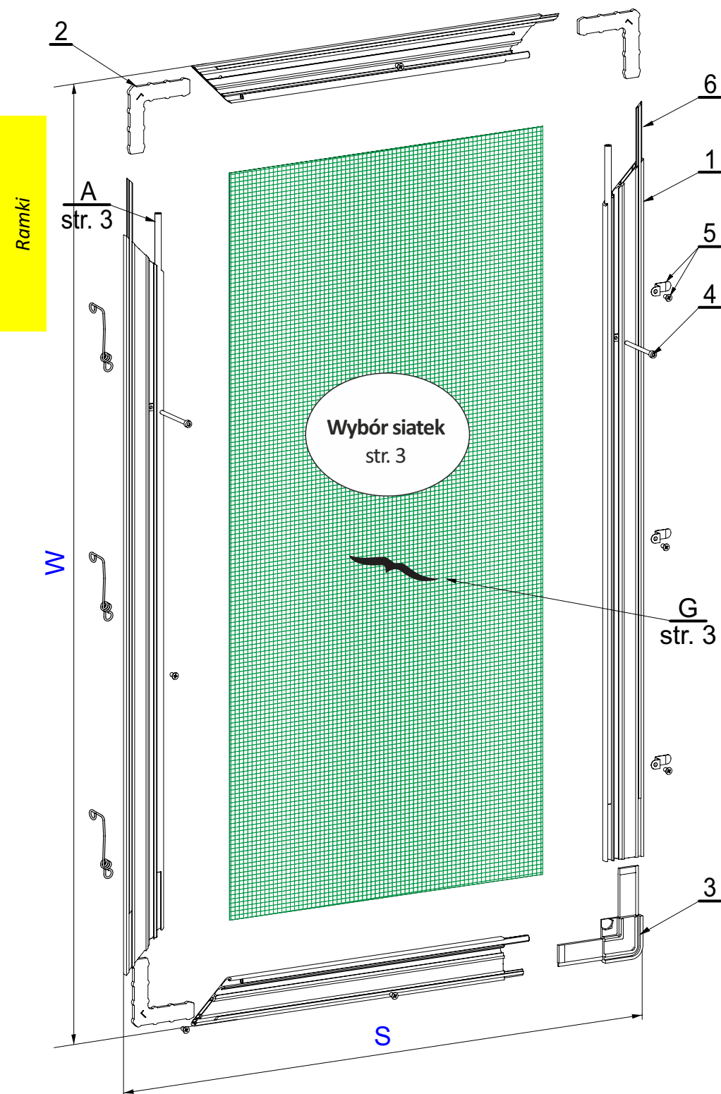
Ramka LICO w oknie
