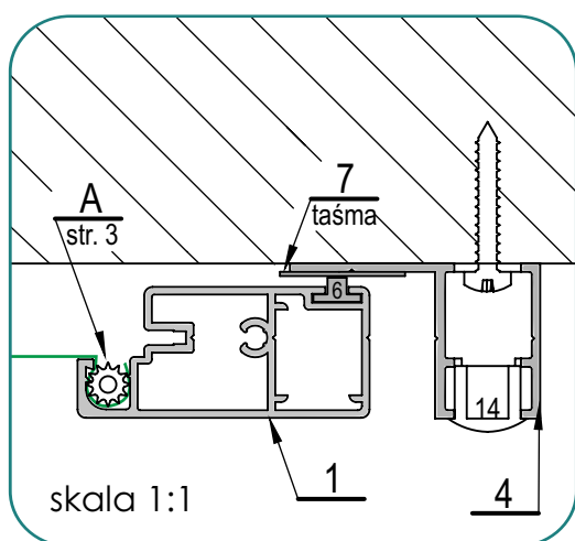
Rama montażowa wraz z listwą magnetyczną
