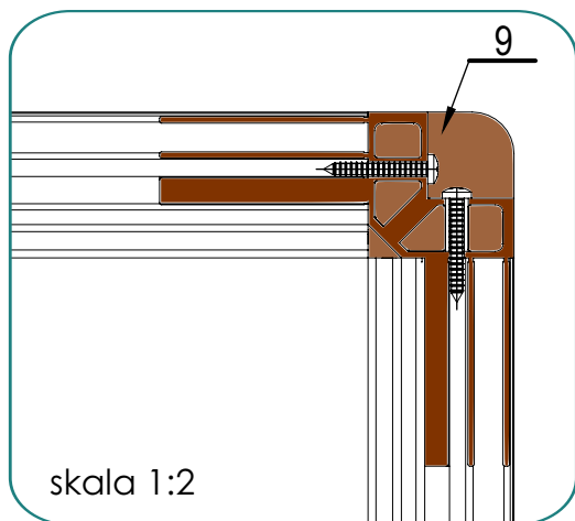
Narożnik zewnętrzny + wkręt
