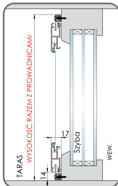
Prowadnica S III u góry i na dole do ramy [mm]
