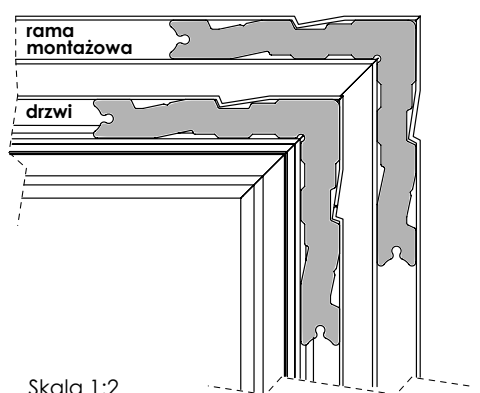
Skala 1:2
